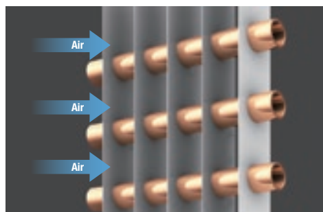
Standardowy wymiennik ciepła
