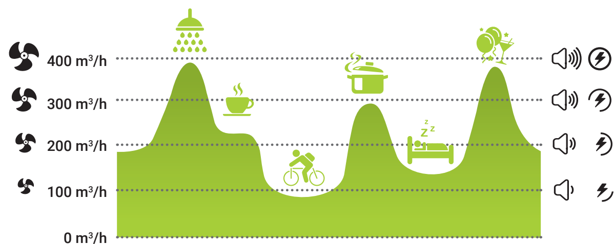
POZIOM PRZEPIYU POWIETRZA Wentylacja regulowana zapotrzebowaniem
